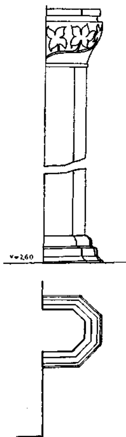
Sl. 5. Profil ulaznog okvira i baze triumfalnog luka u kapeli
