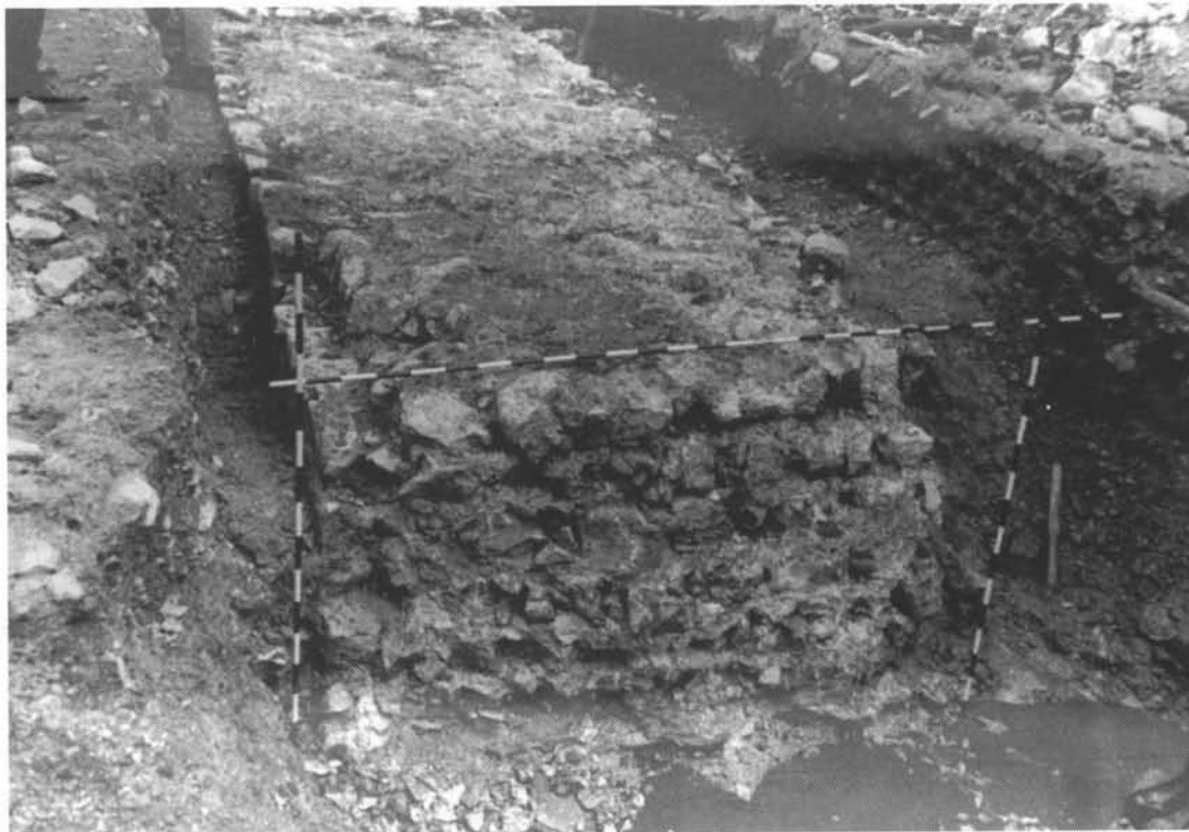
Slika 1. Dio strukture bedema ispod zgrade "Brodmaterijala" u današnjoj Starčevićevoj ulici. Fototeka arheološkog odjela Pomorskog i povijesnog muzeja Hrvatskog primorja, Rijeka 1970.
