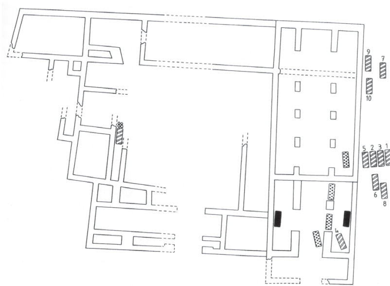
Sl. 2 Biskupija – Crkvina, tlocrt crkve sv. Marije s položajem grobova odličnika (prema Petrinc 2006, 35).
