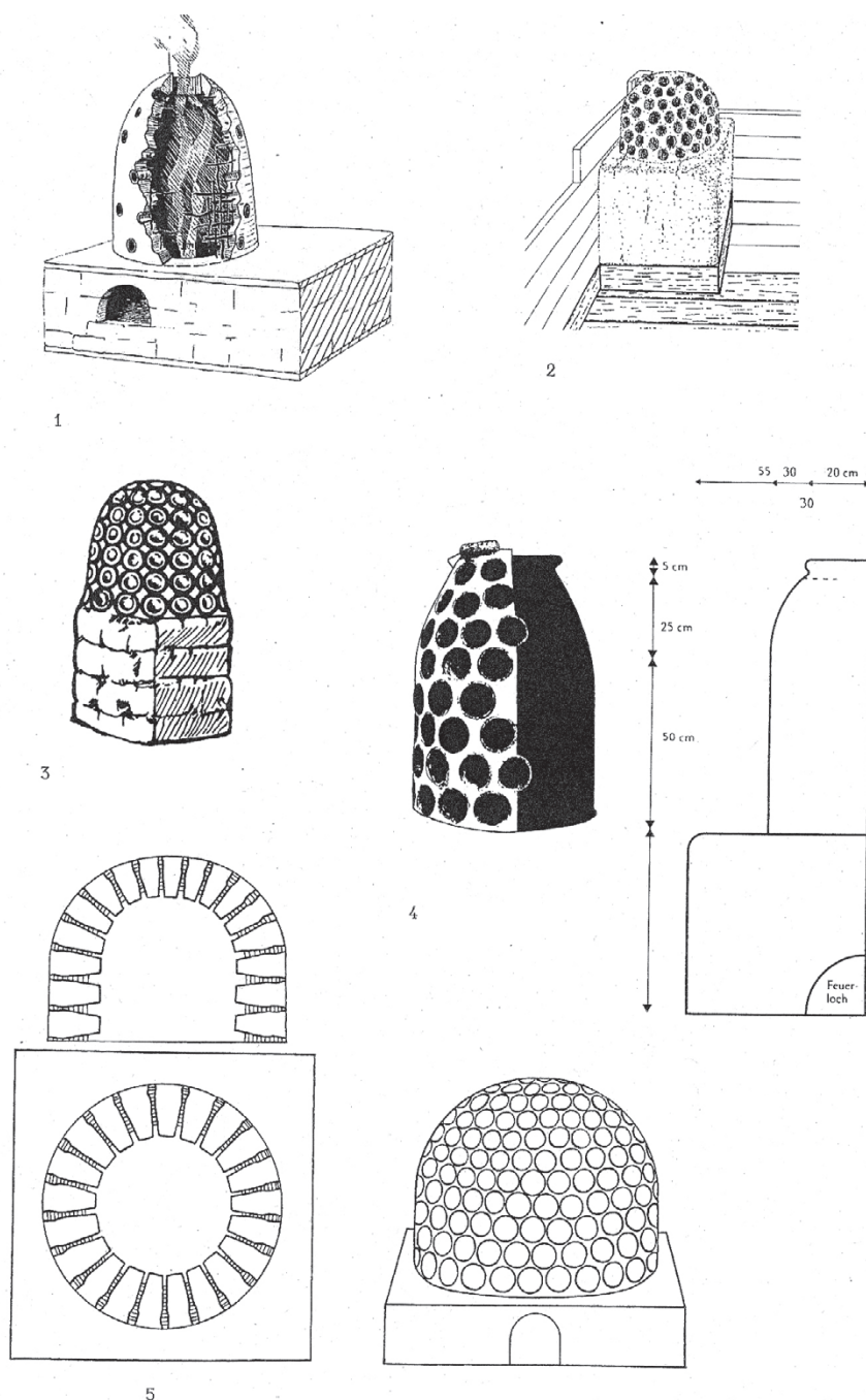
Sl. 1 Rekonstrukcije ranih primjera kaljevih peći: 1. Zürich, Münsterhof, druga četvrtina 13. st.; 2. Winterthur, Metzgasse, 1208. – 1300.; 3. Neuneburg, Freyburg/Unstrut, 13. st., 4. Straubing, Schmidgasse, druga pol. 13. st.; 5. Wiprechtsburg bei Grotzch, 12. st. (prema: Hellenkamp-Lumpe 2006, T. 155).
