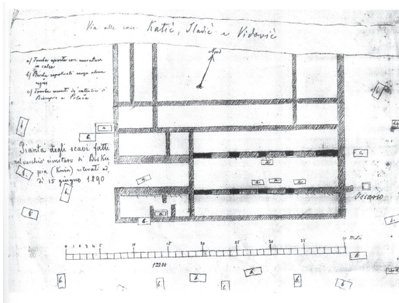
Sl. 1 Biskupija – Crkvina, tlocrt crkve sv. Marije iz 19. st. (prema Milošević 2011, 87).
