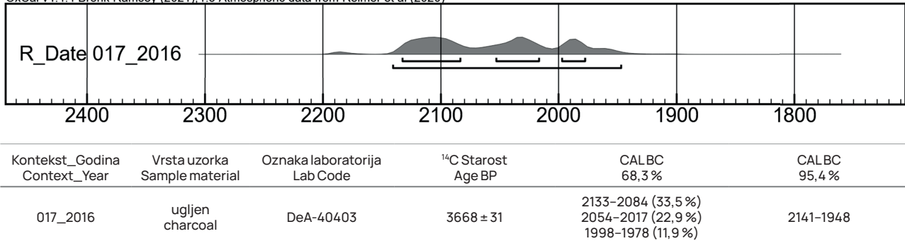
Sl. 3 Radiokarbonski datum za rano brončano doba s nalazišta Kurilovec – Belinščica (prema Molnár 2023). OxCal v4.4.4. (© Bronk Ramsey 2021); IntCal 13 atmospheric curve (Reimer et al. 2020)
